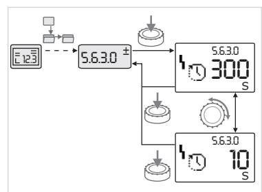
Рис. 38: Настройка с возвратом к элементу меню «Выбор/настройки»
