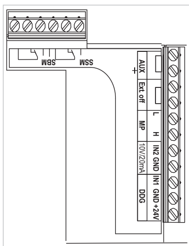
Рис. 25: Клеммы управления
