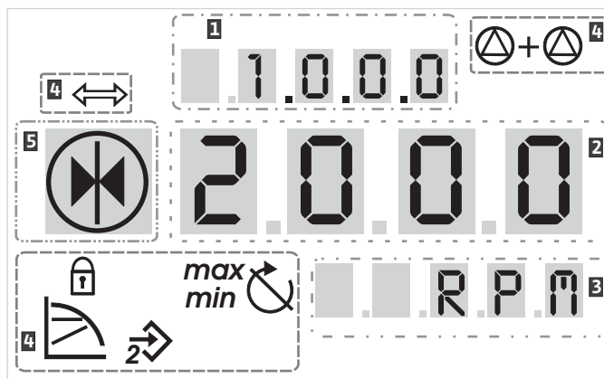
Рис. 30: Структура дисплея
