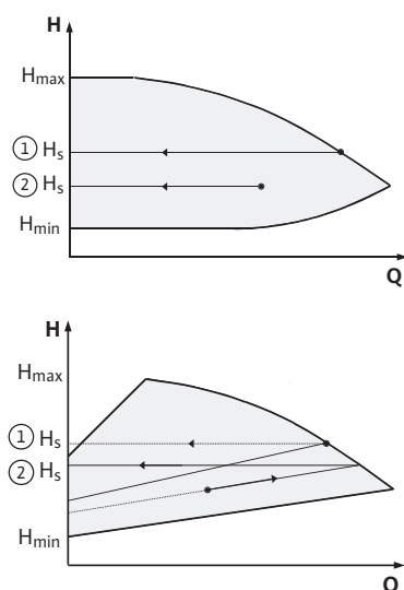
Рис. 43: Регулирование \Delta p -с/ \Delta p -v
