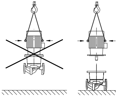
Рис. 20: Транспортировка электродвигателя
