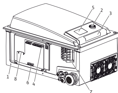
Рис. 9: Электронный модуль
