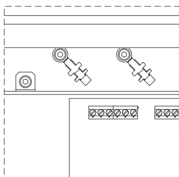
Рис. 24: Экранирование кабелей
