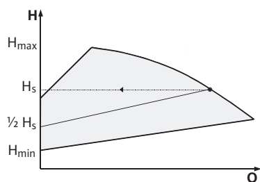
Рис. 11: Регулирование \Delta p-v
